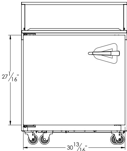
ELEVATION
